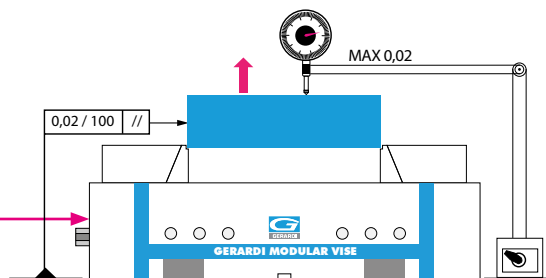
Morsa ancorata con 2 coppie di staffe Art.296 Vise clamped with n. 2 pairs of Art.296
