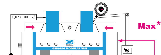
Morsa ancorata con 2 coppie di staffe Art.296 Vise clamped with n. 2 pairs of Art.296
